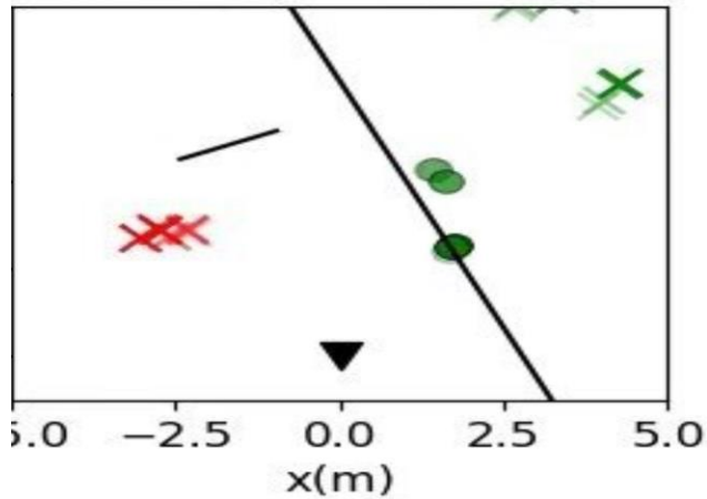
II Estimation(Frame 97)
